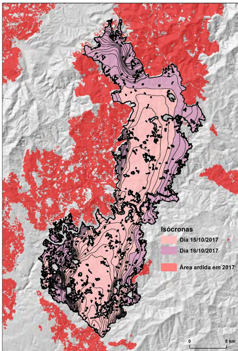
Figura 3.14. Linhas isócronas de propagação do complexo de incêndios de Ponte das Portelhas-Figueiredo-Sertã (1ª ignição) e Nespereira-Pedrogão Pequeno-Sertã (canto sudoeste).
