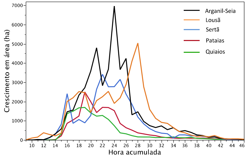
Figura 3.29. Crescimento horário dos mega-incêndios estudados. No eixo das abcissas a hora acumula desde as 9 horas do dia 15 de outubro.
