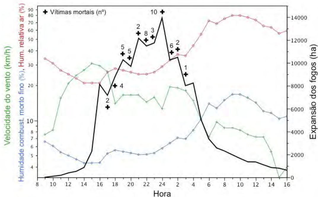
Figura 1. Evolução horária da expansão dos mega-incêndios estudados (Pataias, Quiaios, Lousã, Sertã e Arganil-Seia), ocorrência de vítimas fatais e condições piro-meteorológicas (estação do IPMA em Viseu) das 9 horas do dia 15 de outubro às 16 horas do dia 16 de outubro de 2017. Foi selecionada a estação de Viseu porque revela simultaneamente o efeito Ophelia no vento e o downdraft após a meia noite.
