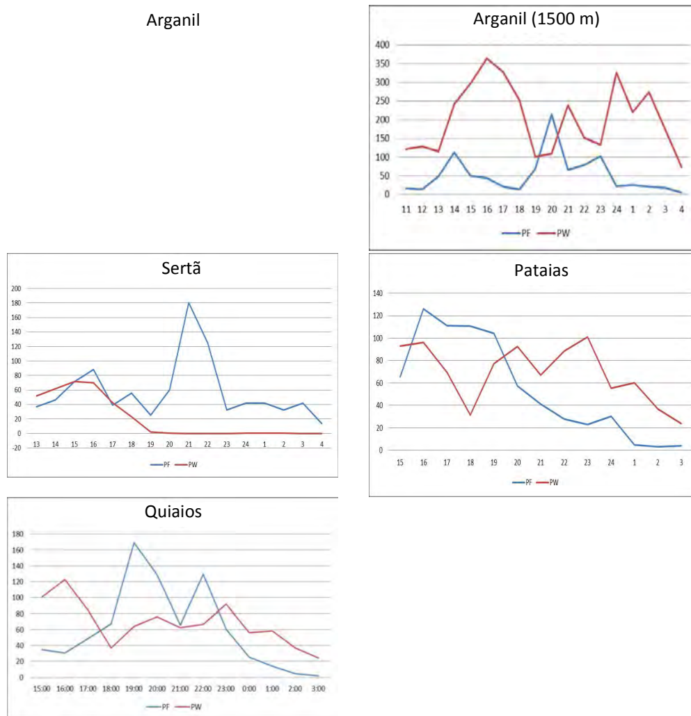
Figura 3.30. Evolução da relação entre a potência do vento (Pw) e a potência do fogo (Pf) para quatro dos incêndios. No caso do complexo de Arganil-Seia apresenta-se também a relação a 1500 m de altitude; note-se o domínio de Pf cerca das 20 horas, momento de PyroCb e downdraft nesse incêndio.
