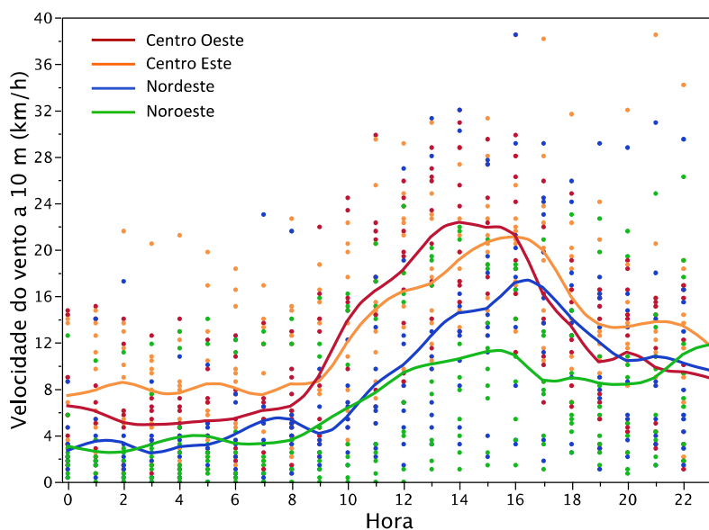
Figura 3.6. Médias horárias (UTC) da velocidade do vento (a 10 m de altura) para as estações meteorológicas do IPMA no Centro e Norte do país, 15 de outubro de 2017. As linhas representam splines cúbicos ajustados ao conjunto de estações de cada uma das regiões consideradas.
