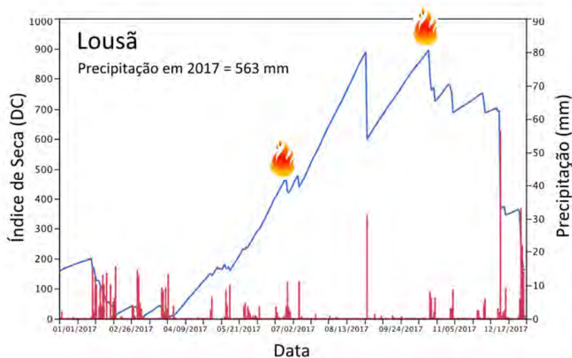
Figura 3.1. Precipitação observada e Índice de Seca (DC) na estação meteorológica do IPMA no aeródromo da Lousã durante o ano de 2017. As chamas assinalam os dois piro-eventos catastróficos.
