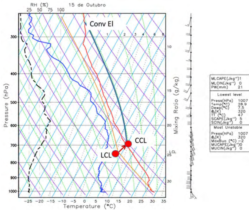
Figura 3.18. Radiosondagem sobre Lisboa, 15 de outubro de 2017.
