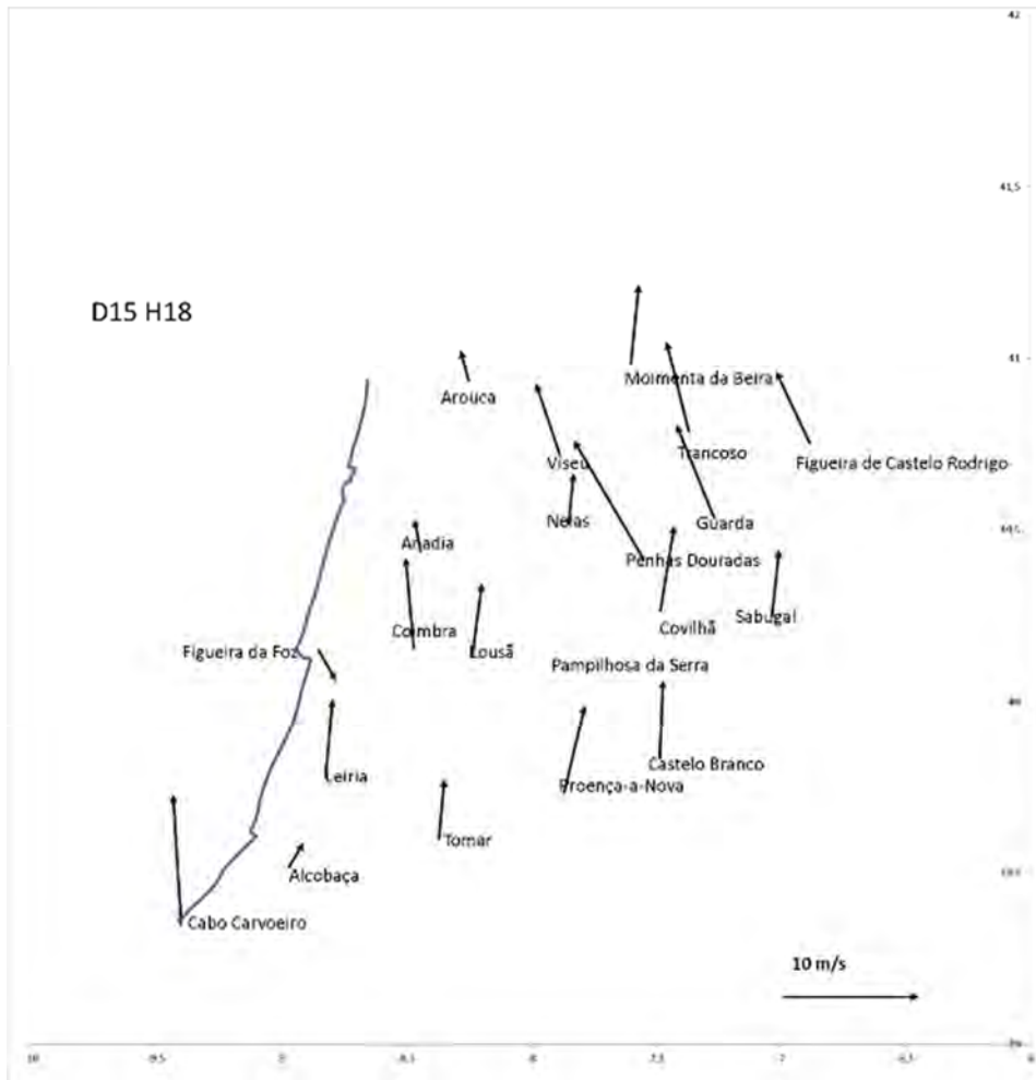
Figura 3.32. Campo de ventos do dia 15 de outubro às 18:00 horas. A estação da Figueira da Foz é a única discordante e aponta ao quadrante sul.
