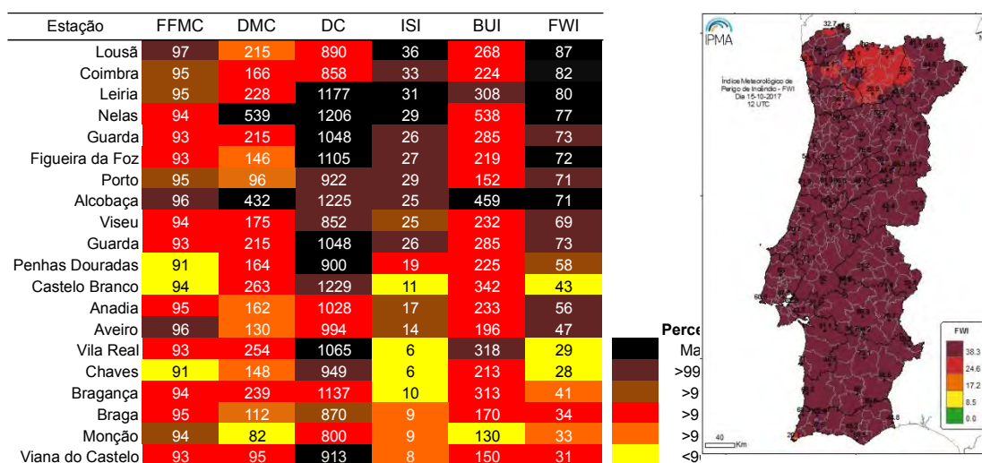
Figura 3.8. Índices do Sistema Canadano de Perigo Meteorológico de Incêndio (FWI) observados no dia 15 de outubro de 2017 em estações meteorológicas selecionadas (IPMA): valores e percentis (período 2001-2016) e mapa de classificação do nível de perigo.
