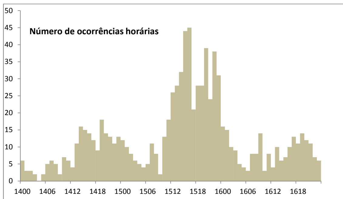
Figura 2.7 Evolução horária do número de ocorrências observadas nos dias 14 a 16 de outubro de 2017 (colunas a cheio). Os quatro algarismos no eixo horizontal representam o dia e a hora.
