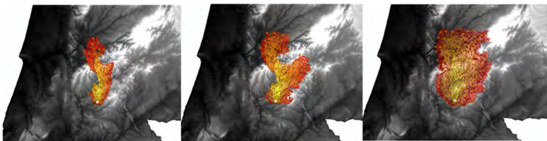
Figura 3.35. Simulação do incêndio da Sertã, ajustada à realidade (esquerda) e projetada para 48 horas (centro), e simulação livre (condições do dia 15 de outubro durante 48 horas) se o incêndio tivesse ocorrido sem que os incêndios de junho e agosto tivessem sucedido.
