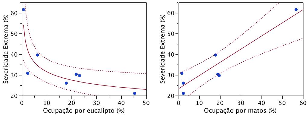
Figura 3.36. Relação entre a área ardida com severidade Extrema (% do total) e a ocupação do solo por eucalipto ( R^2=0,76 , p=0,0109 ) e por matos ( R^2=0,76 , p=0,0027 ) para os mega-incêndios individuais.
