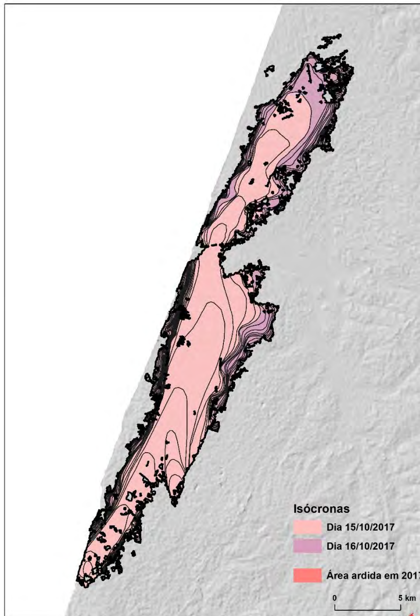
Figura 3.15. Linhas isócronas de propagação do complexo de incêndios de Légua-Pataias (1. a ignição, extremo sul) e Burinhosa-Pataias (2. a ignição).
