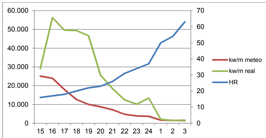
Figura 3.24. Intensidade real e modelada do incêndio de Burinhosa-Pataias das 15 horas do dia 15 de outubro às 3 horas do dia 16 de outubro. Repare-se na evolução da humidade do ar (HR).
