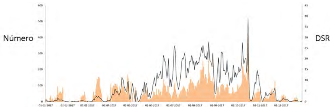
Figura 2.2 Evolução ao longo do ano de 2017 do número de ocorrências (colunas a cheio e escala no eixo vertical à esquerda) e do valor do índice DSR ("Daily Severity Rating") do Sistema Canadano de Indexação do Perigo de Incêndio (linha a preto e escala no eixo vertical à direita). O número de ocorrências mais elevado (495) corresponde ao dia 15 de outubro em que ocorre igualmente o valor de DSR mais elevado (38,7).
