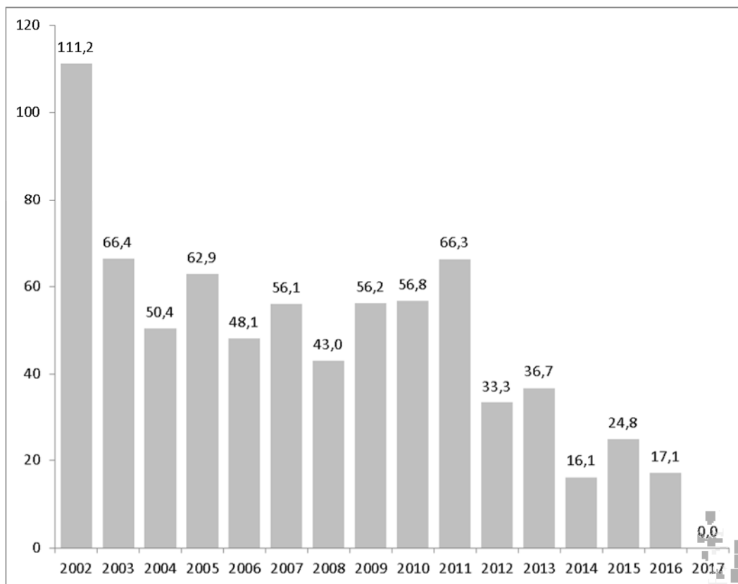
Figura 2.3 Valores do fator Ano a incluir no modelo de previsão ( \alpha_{\text{Ano}} ) que indicam que o número de ocorrências tem vindo a diminuir ao longo dos anos: o número diário de ocorrências era em média mais 111,2 em 2002 do que em 2017.
