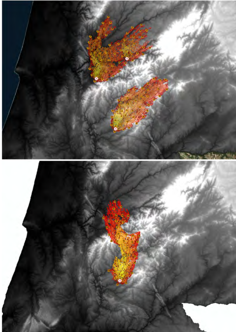
Figura 3.32. Simulação sem interação do conjunto Lousã e Arganil-Seia (norte) e Sertã (sul), imagem superior. Observe-se como o fogo da Sertã se dirige para NE, o que não aconteceu na realidade. A simulação na imagem inferior é corrigida com os valores meteorológicos da Lousã assumindo que devido ao indraft estavam a afetar o incêndio a sul.
