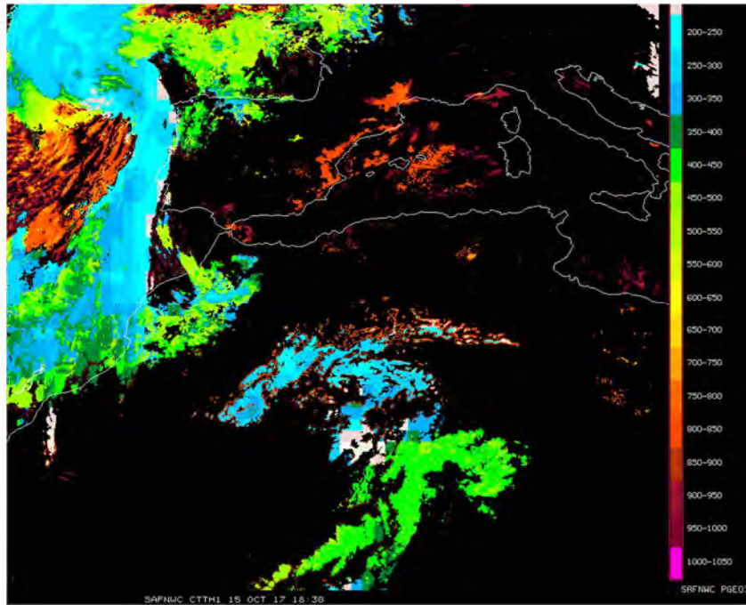
Figura 3.22. Imagem Meteosat do topo de nuvens em 15 de outubro de 2017, presente às 17 horas UTC até 9 km de altitude (cima) e ausente às 18:30 horas UTC (baixo).
