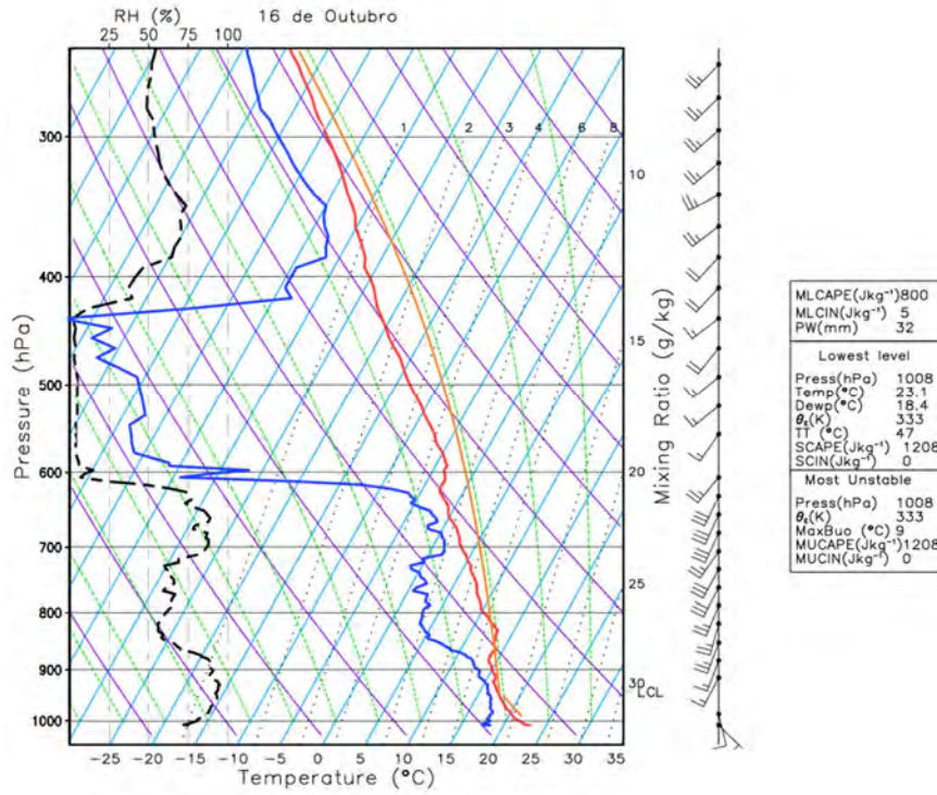
Figura 3.19. Radiosondagem sobre Lisboa, 16 de outubro de 2017.
