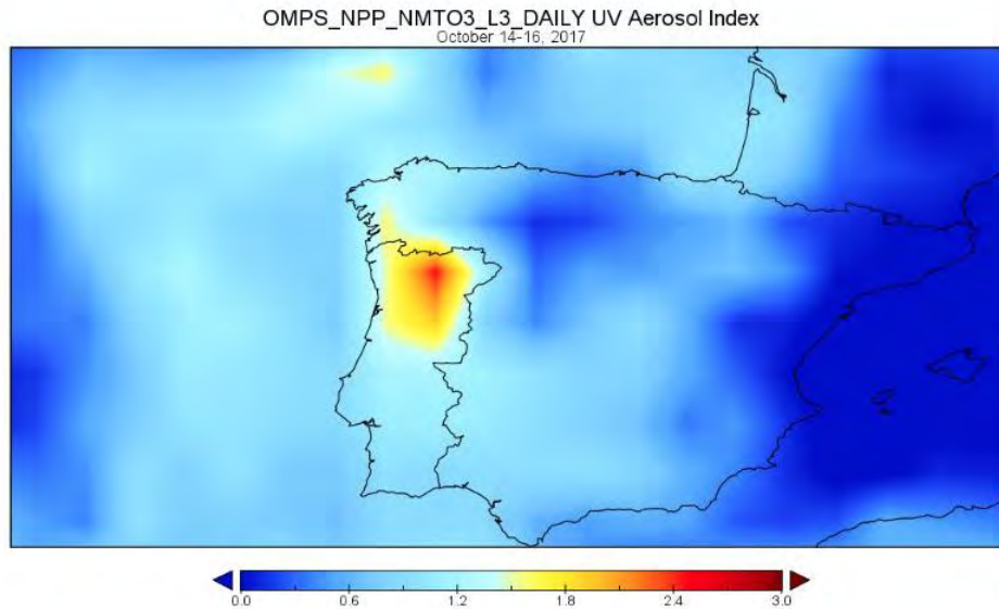
Figura 3.28. Índice de aerossol medido pelo satélite Suomi NPP, com valores elevados no Norte de Portugal e sobre a zona de ventos fracos que são indicativos das plumas de fumo dos incêndios. A concentração elevada de fumo dos incêndios, porém sem dispersão, confirma a piro-convecção.
