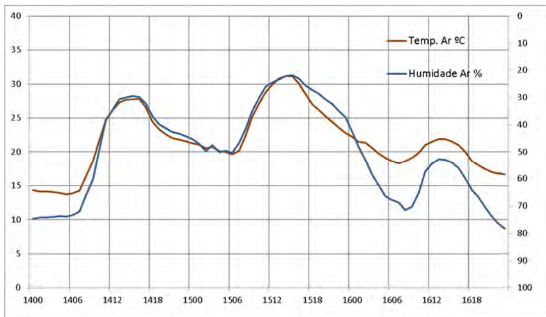
Figura 2.8 Evolução horária das médias das temperaturas e humidades relativas do ar para as 24 estações meteorológicas da região durante os dias 14 a 16 de outubro de 2017. No eixo dos Y à esquerda estão representadas as temperaturas do ar (°C) e à direita, em ordem inversa, as humidades relativas do ar (%). De registar a grande relação (inversa) entra as duas variáveis meteorológicas. Os quatro algarismos no eixo horizontal representam o dia e a hora.
