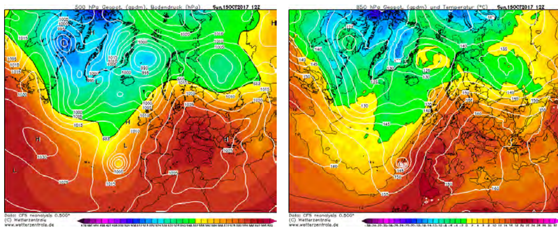
Figura 3.4. Cartas sinóticas para o dia de 15 de outubro de 2017.
