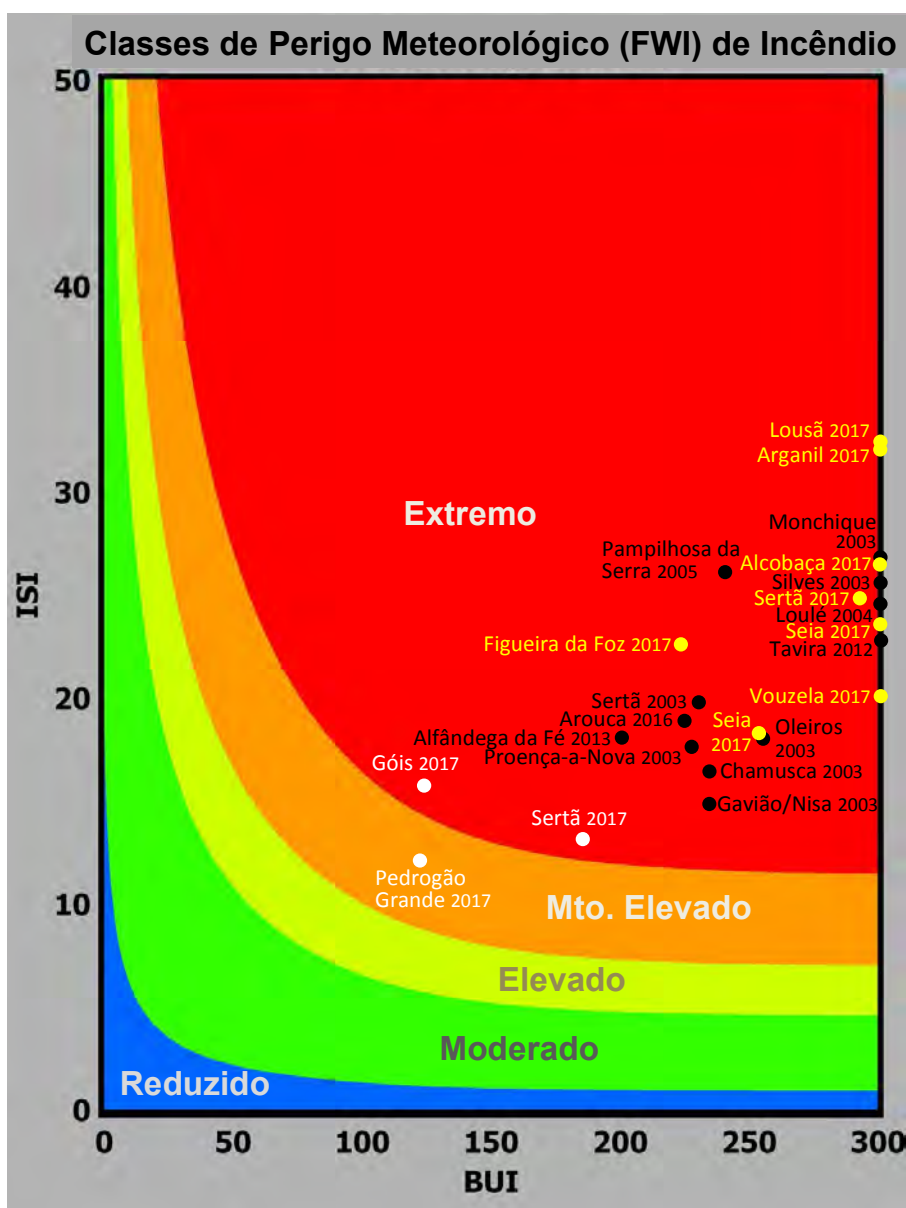
Figura 3.9. Classificação do perigo meteorológico de incêndio, incluindo índices de velocidade de propagação do fogo (ISI) e de disponibilidade de combustível (BUI) do sistema FWI, associado aos mega-incêndios (>10 000 ha) ocorridos em Portugal. A amarelo os incêndios do dia 15 de outubro de 2017, a branco os restantes mega-incêndios de 2017. O índice ISI respeita às 12UTC e, portanto, não reflete as
