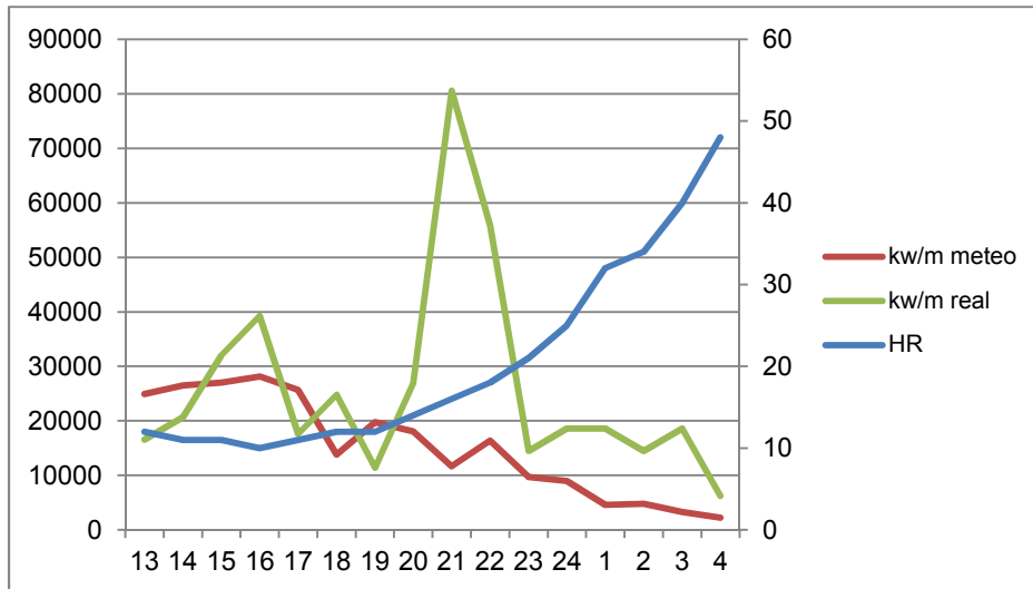
Figura 3.25. Intensidade real e modelada do incêndio de Figueiredo-Sertã das 15 horas do dia 15 às 4 horas do dia 16 de outubro. Repare-se na evolução da humidade do ar (HR).
