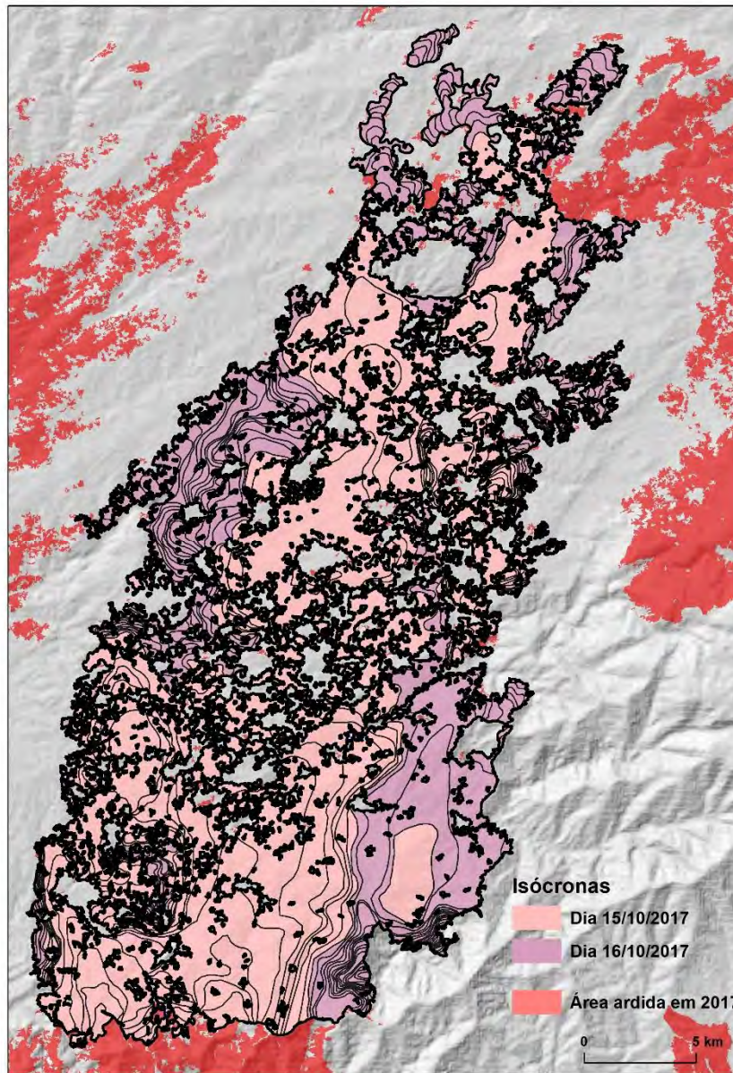
Figura 3.13. Linhas isócronas de propagação do complexo de incêndios de Sandomil-Seia (1ª ocorrência, sector centro-leste), Esculca-Côja-Arganil (2ª ocorrência, com duas ignições junto ao limite sul) e Vide-Seia (3ª ocorrência, sudeste).
