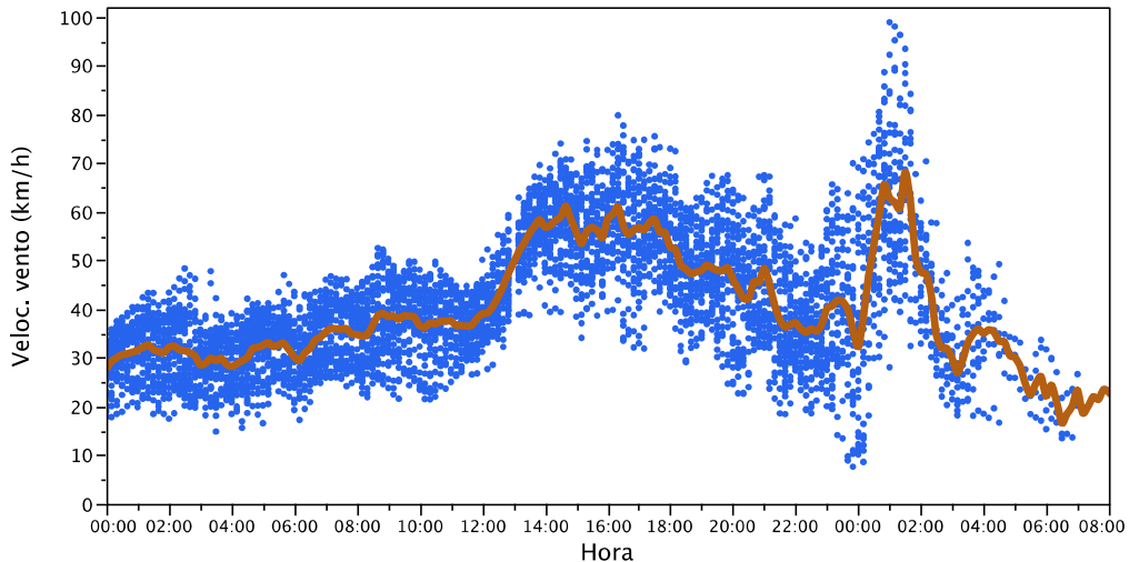
Figura 3.27. Velocidade do vento (médias de 10 minutos) ao nível das turbinas no parque eólico de Fajão, Pampilhosa da Serra, durante o dia 15 de outubro e até às 8 horas do dia 16 de outubro de 2017. A linha resulta de um spline cúbico ajustado ao conjunto de observações individuais. Veja-se a redução que antecede os valores máximos registados durante o período.
