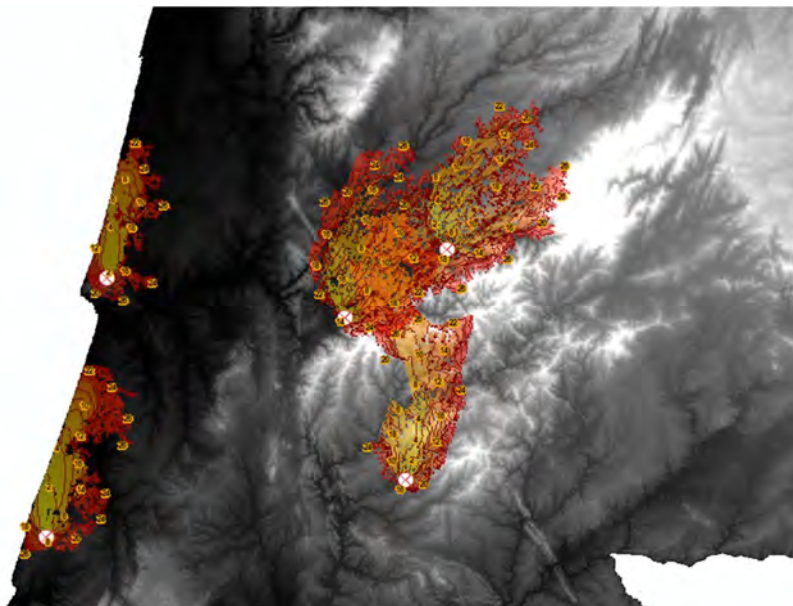
Figura 3.33. Simulação ajustada dos 5 incêndios estudados mostrando o seu crescimento máximo possível durante 26 horas.
